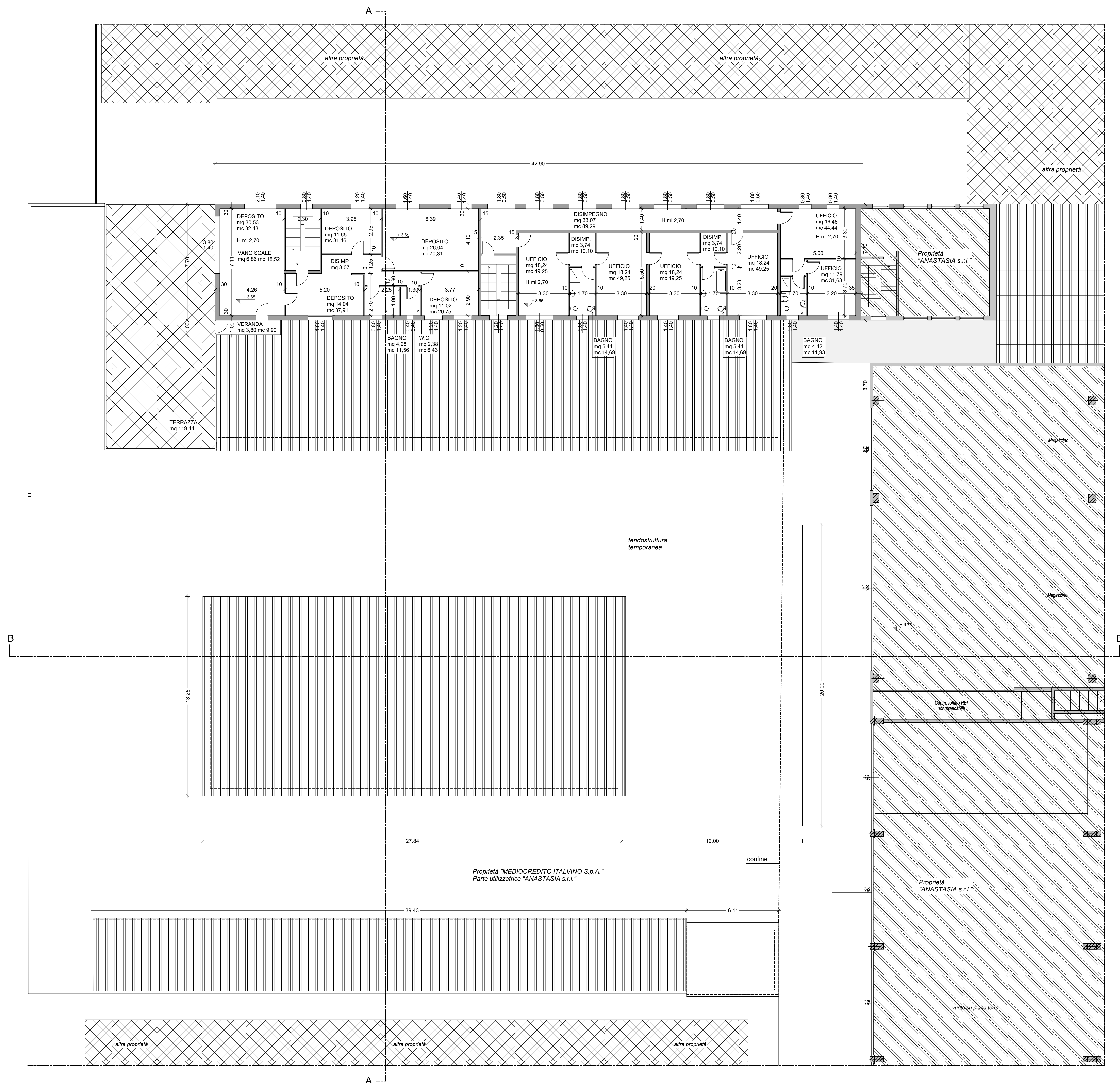
STATO DI FATTO PIANTA PIANO PRIMO scala 1:100
